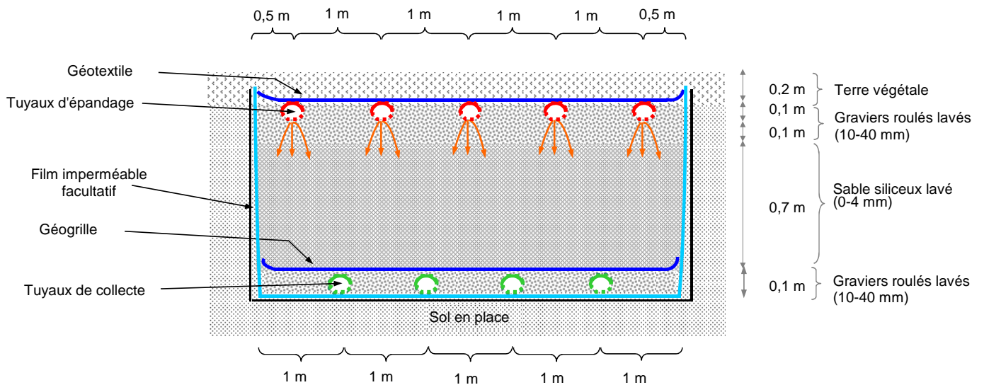
TUYAU D'EPANDAGE
