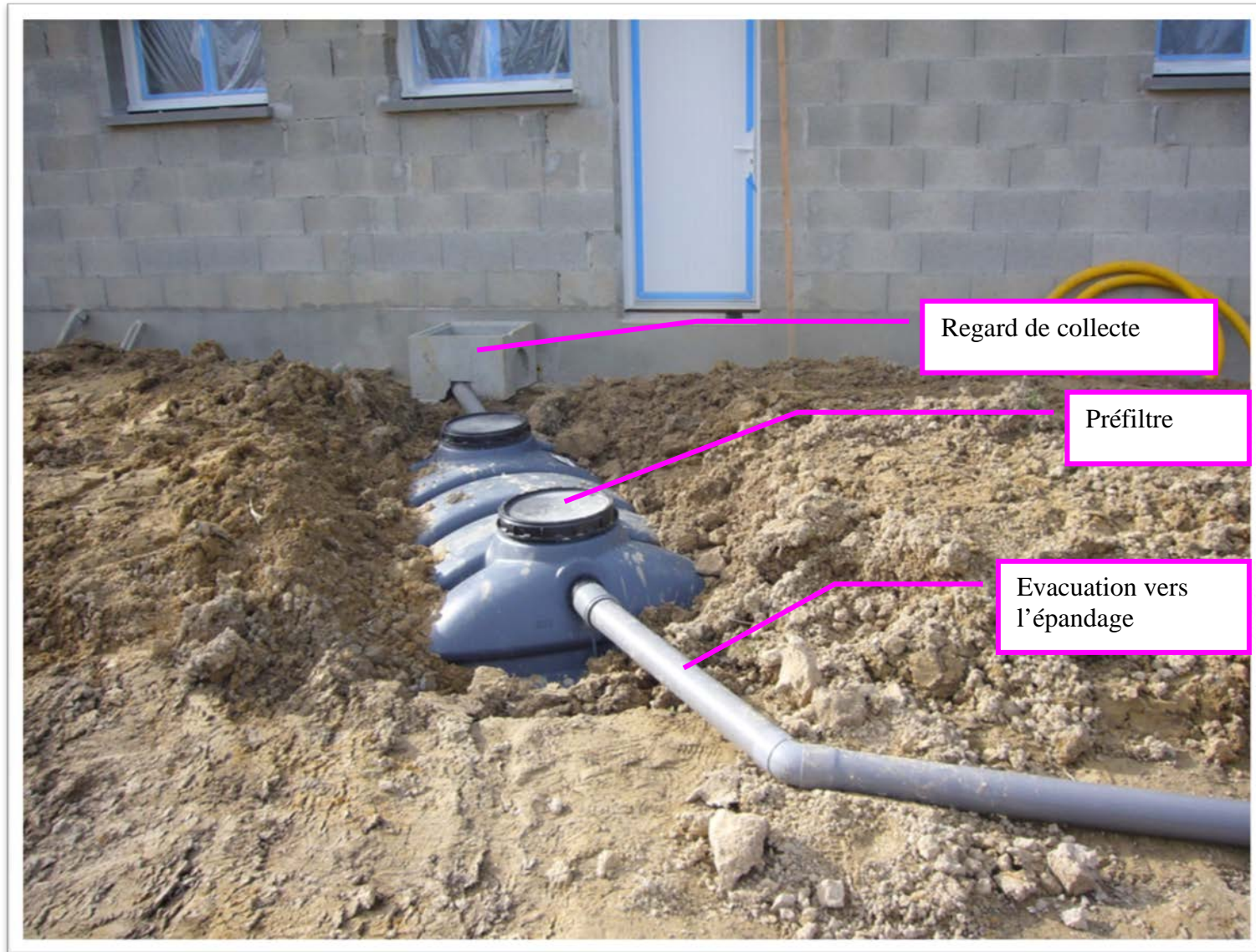
Fosse en plastique avec préfiltre intégré
